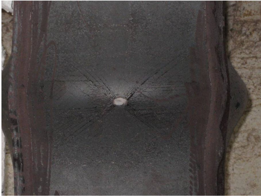
照片3：試驗後試體破壞情況(III)
