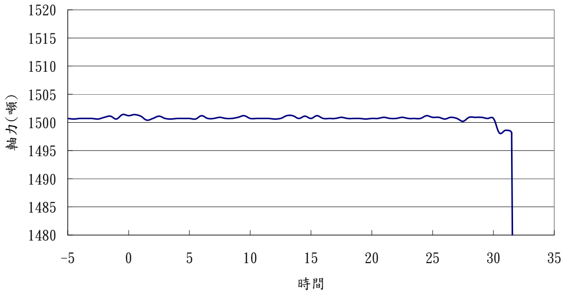
圖 6 加載歷時曲線圖
