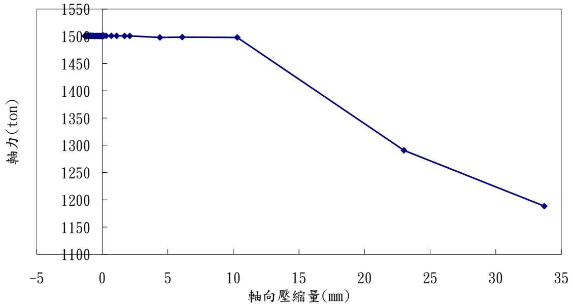
柱軸力與壓縮量歷時
