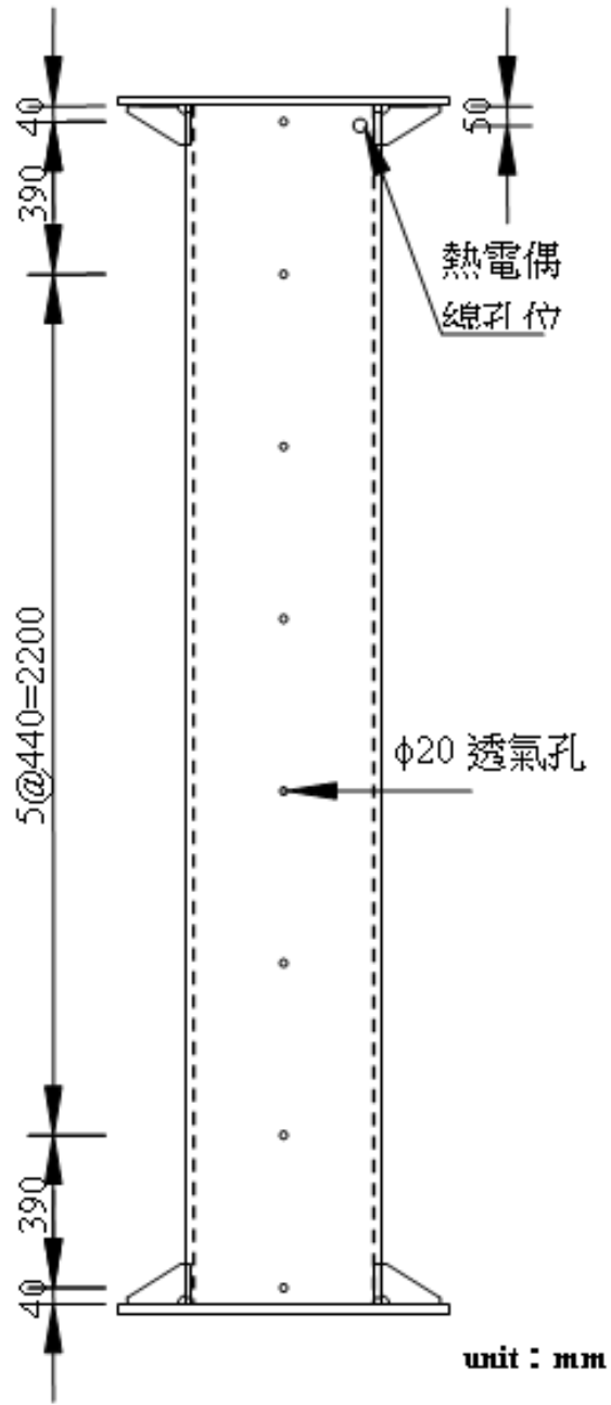
圖 3 試體立面圖
