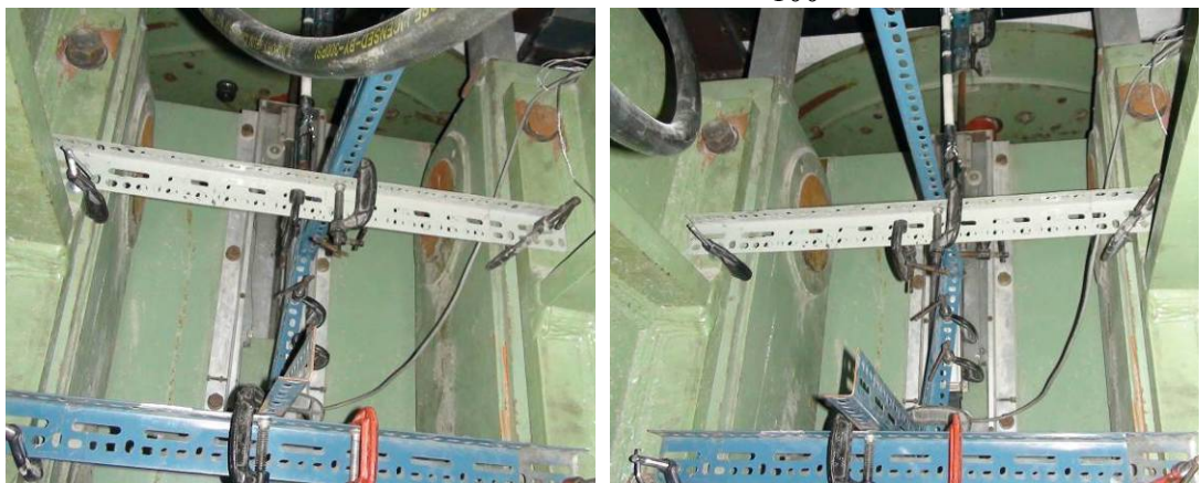
圖 7 壓縮量測點位置圖
