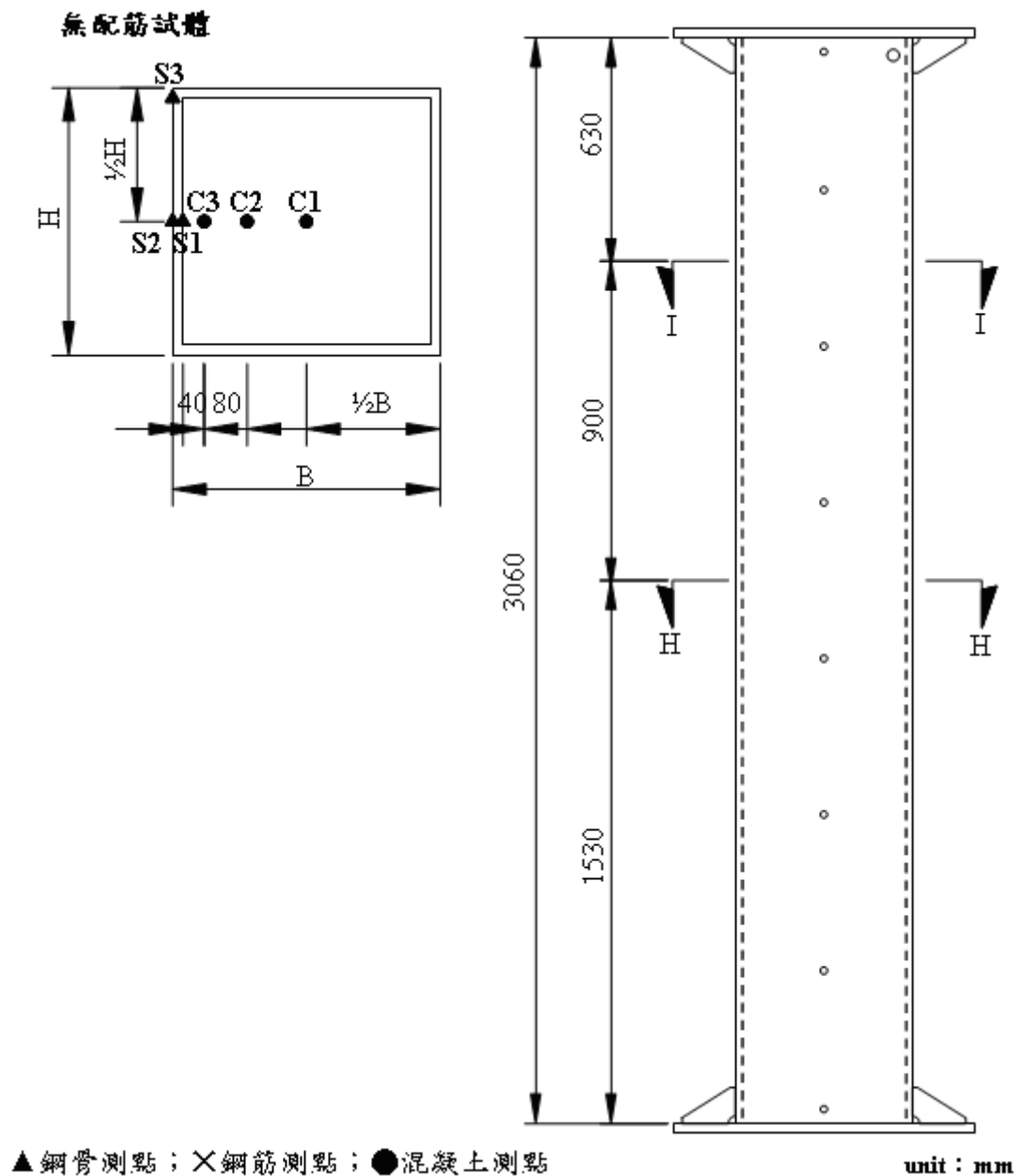
圖5 試體溫度測點分布圖
