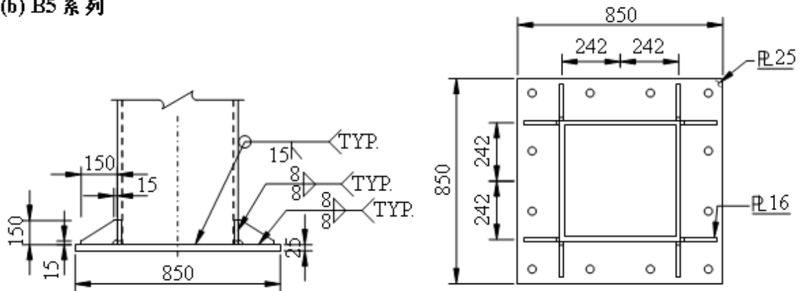
圖2 柱底端板
