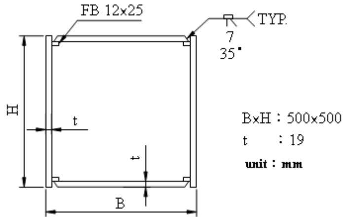
圖1 試體斷面
