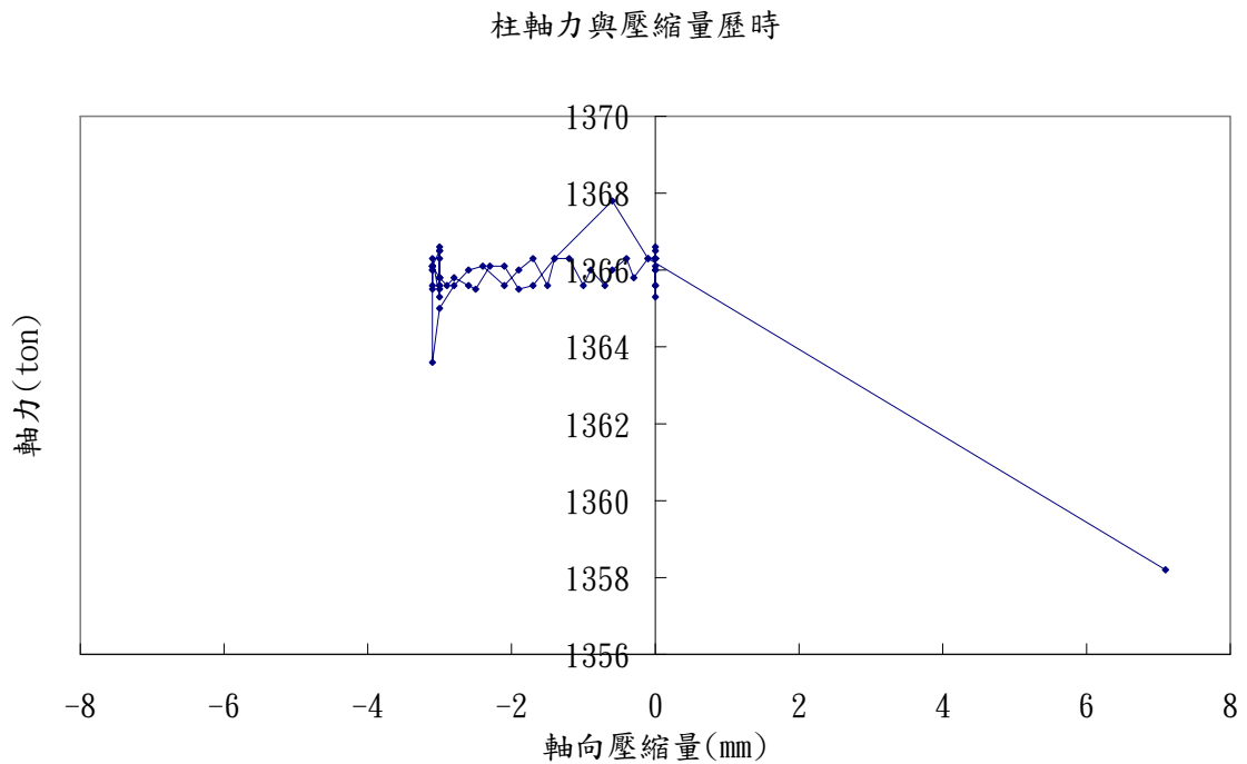
圖 10 軸力與軸向壓縮量歷時曲線圖
